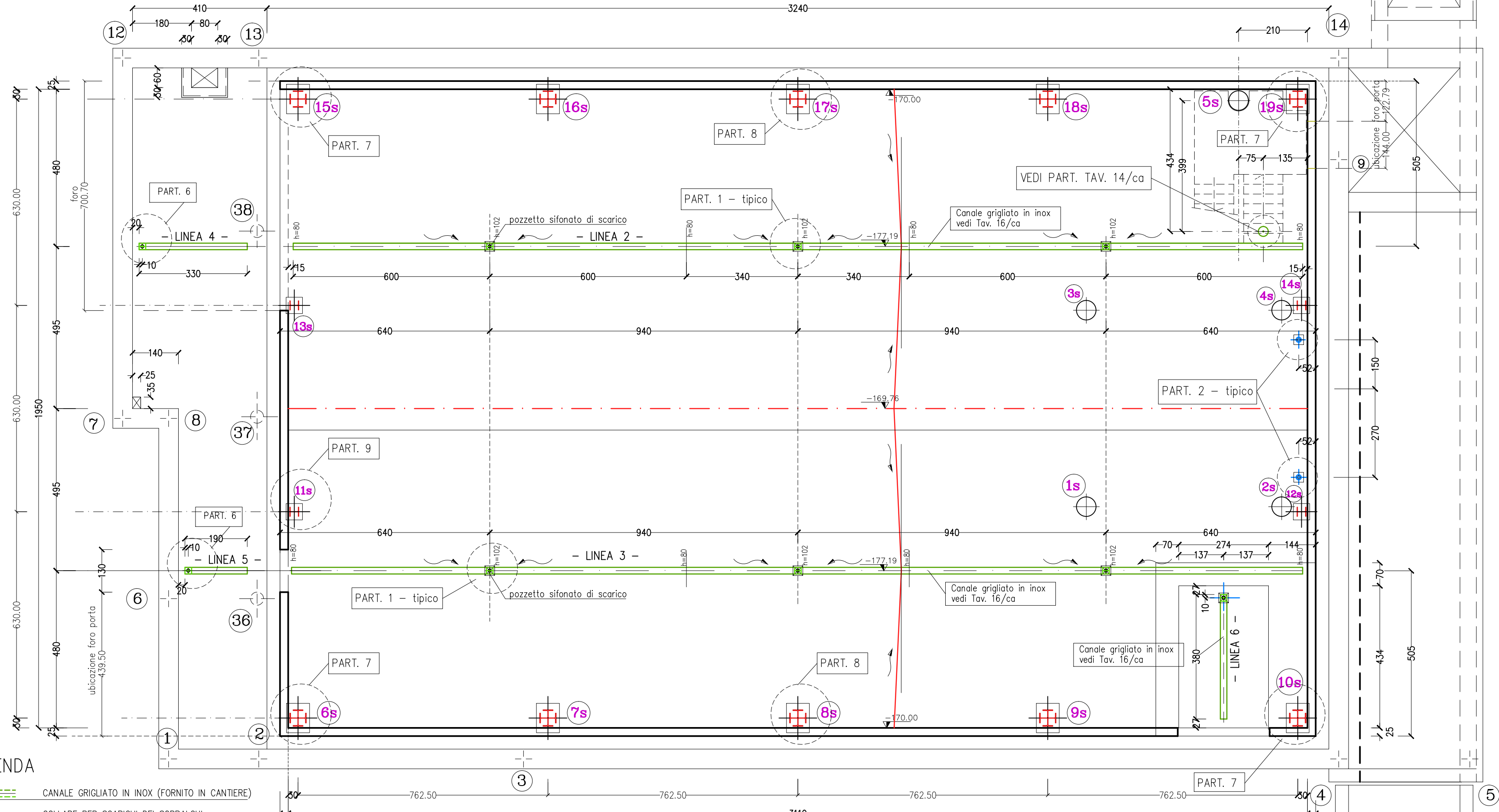
PIANTA -170.00 -SCARICHI ED INOX scala 1:100
