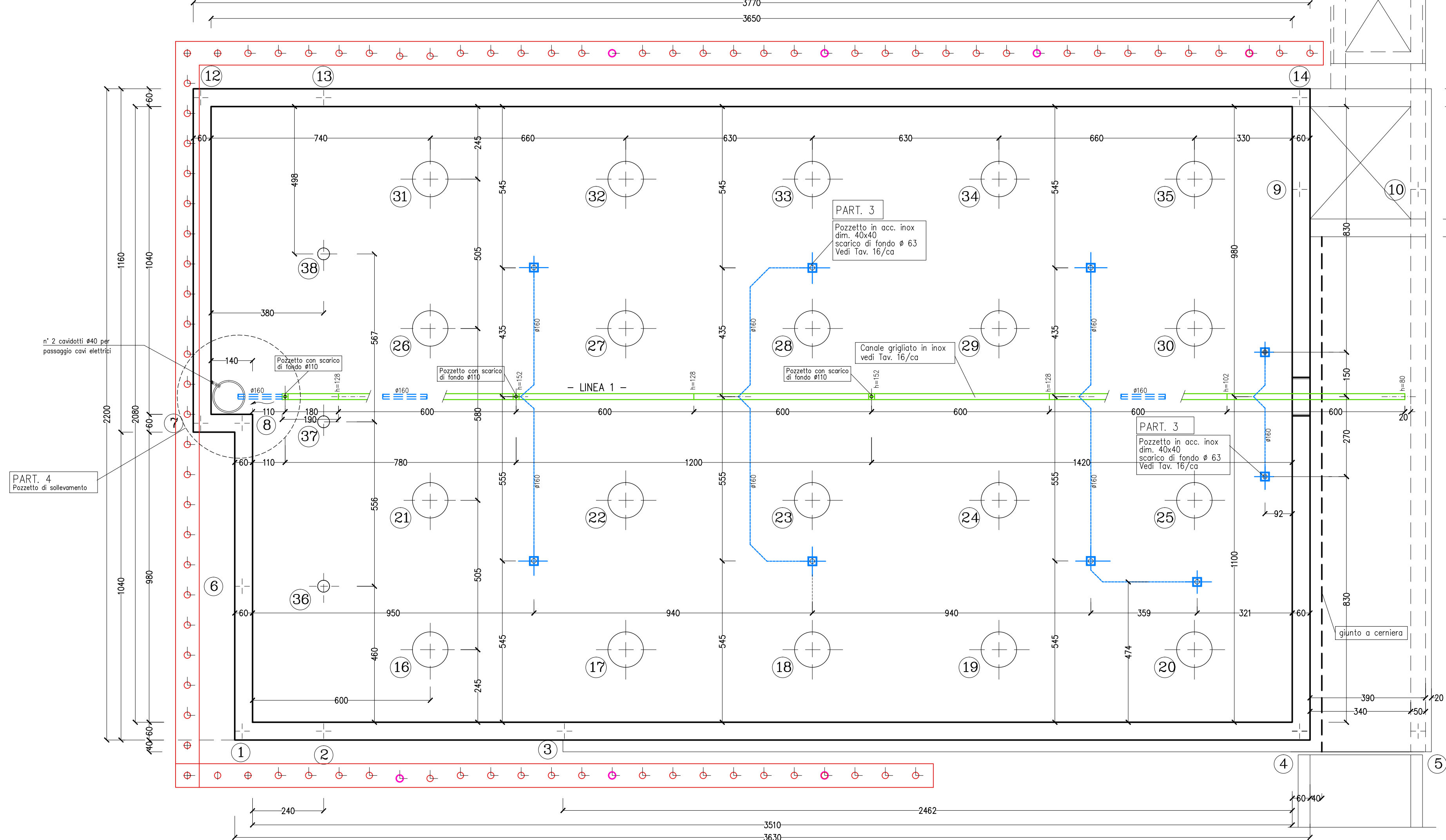
PIANTA -530.00 -SCARICHI ED INOX scala 1:100
